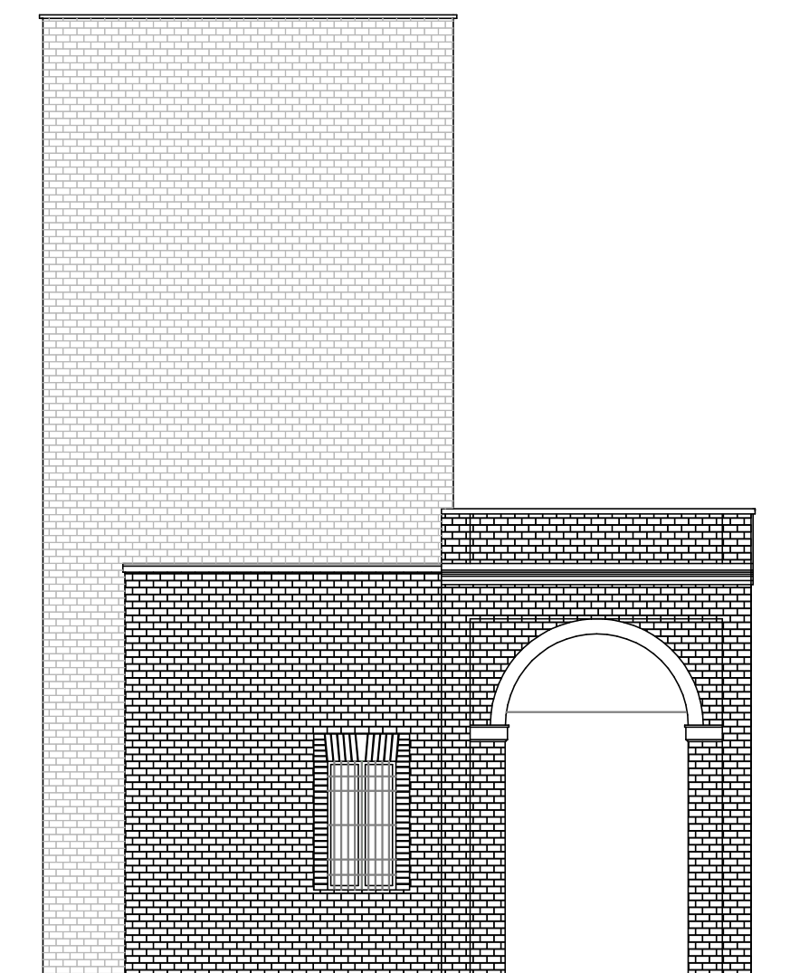
PROSPETTO AD OVEST
