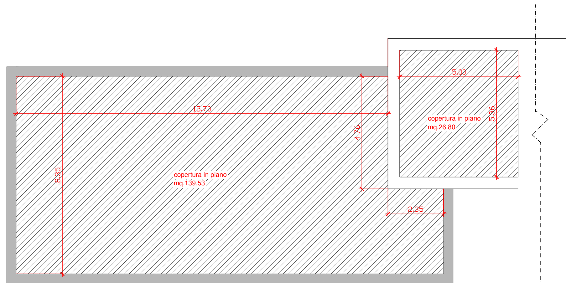
COPERTURA LOCALI COMUNALI E LOGGIATO
