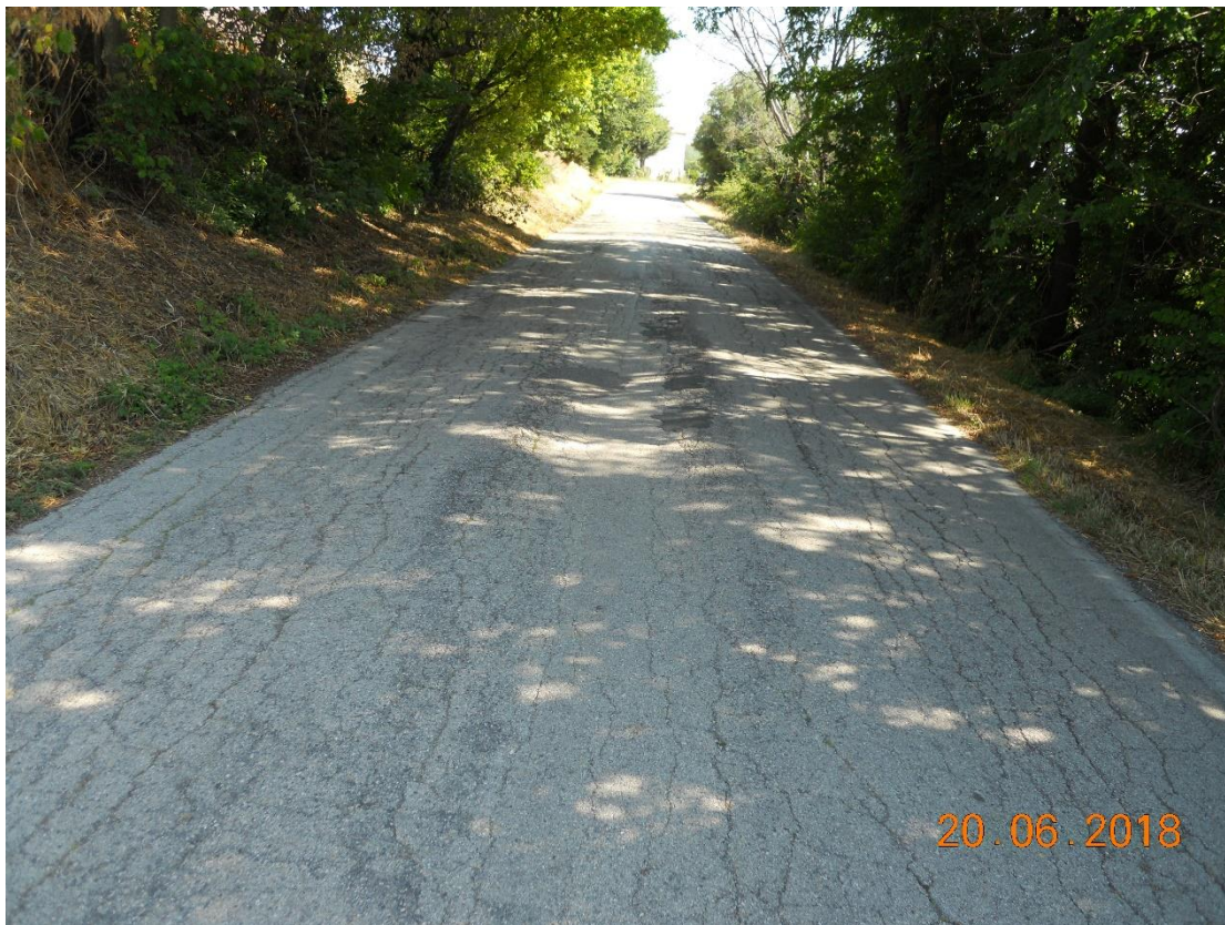
Foto 5. Km 6+000 - Fessurazione a ragnatela della pavimentazione stradale.
