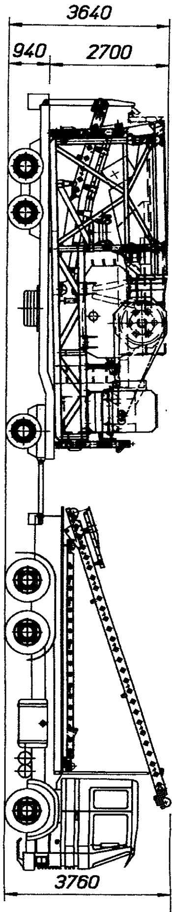
fig. 11 - macchina in assetto da trasporto su autotreno
